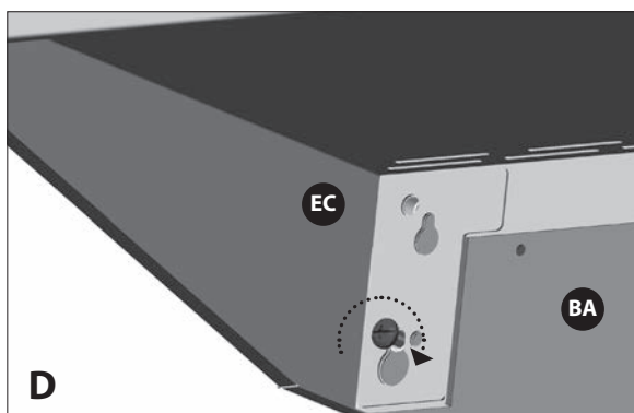
D Vue arrière dessous la tablette latérale gauche
