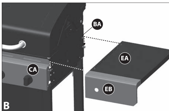
B Vue latérale droite
