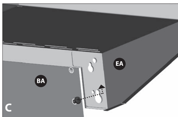
C Vue arrière dessous la tablette latérale droite
