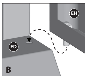
Vue rapprochée du bas de la porte
