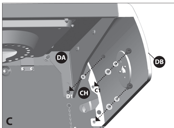
C Avant, vue latérale gauche
