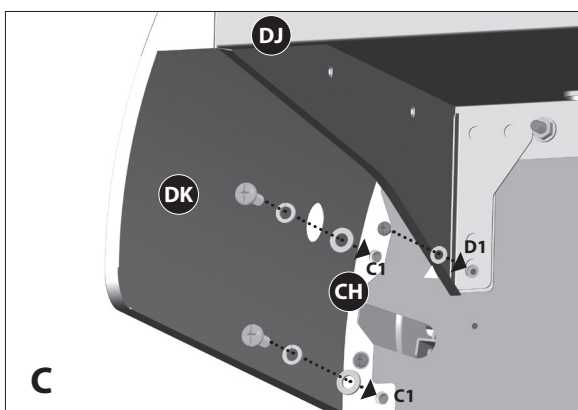
Vue dessous la tablette latérale droite
