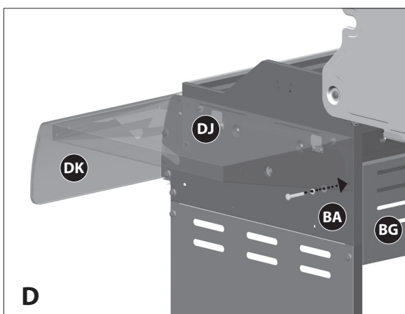
Arrière, vue latérale droite
