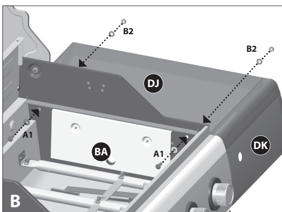
Vue de l'intérieur du boîtier des brûleurs
