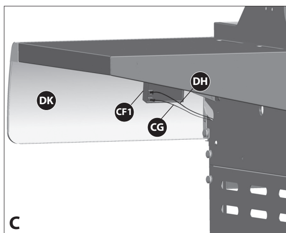
C Vue dessous la tablette latérale droite
