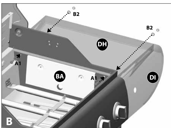
Vue de l'intérieur du boîtier des brûleurs
